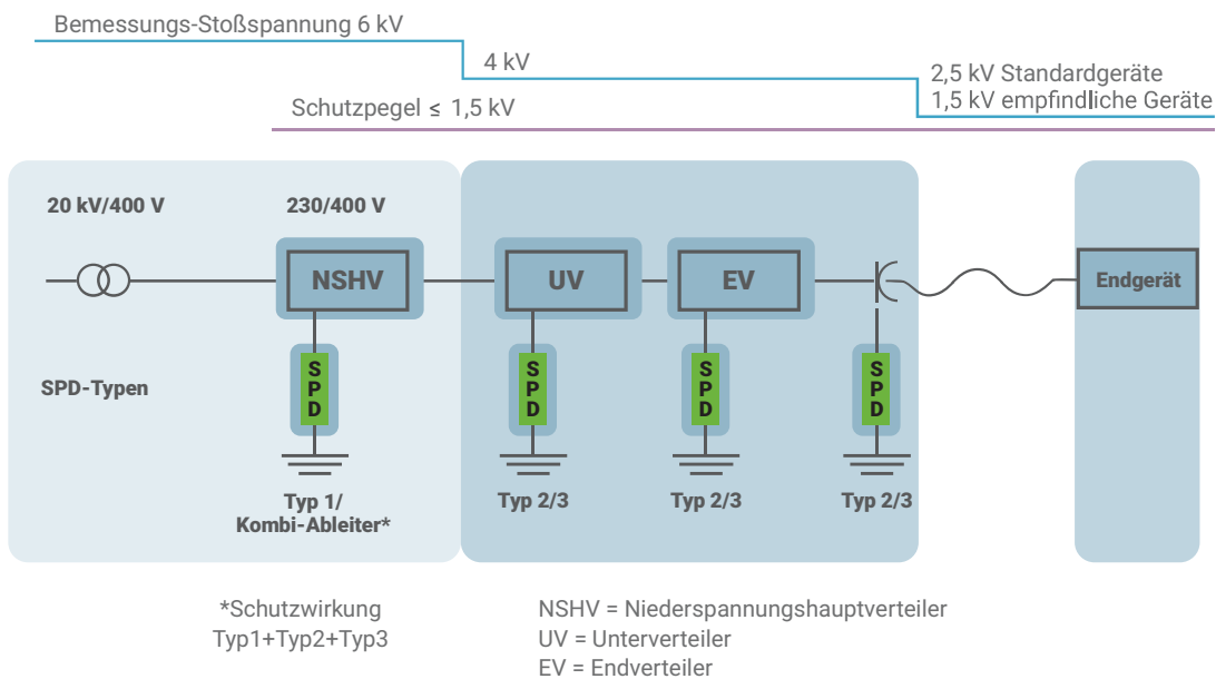
> Bild 8: Zusammenhang Bemessungs-Stoßspannung und Schutzpegel
