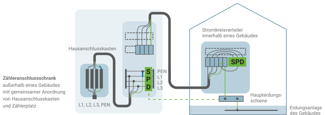
> Bild 15: Beispiel für Überspannungsschutz im Hauptstromversorgungssystem bei Zähleranschlusschrank außerhalb eines Gebäudes und Betriebsmittel eines intelligenten Messsystems im Zähleranschlusschrank
