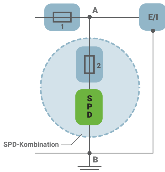
> Bild 1: SPD-Kombination
