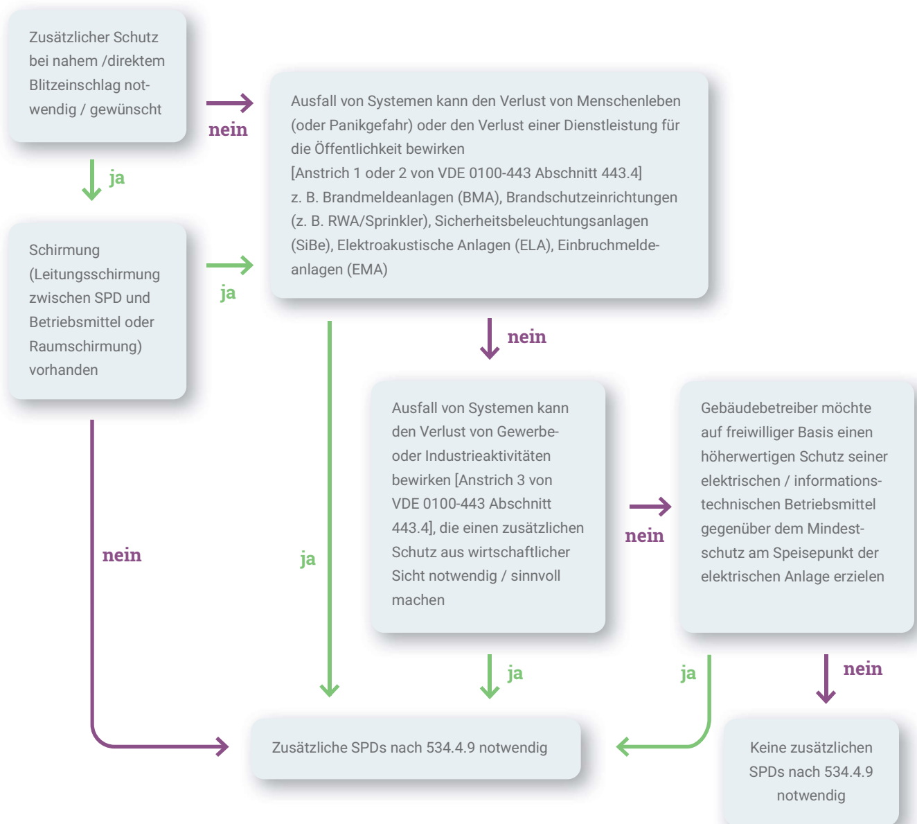
> Bild 7: Entscheidungshilfe zur Notwendigkeit von zusätzlichen SPDs
